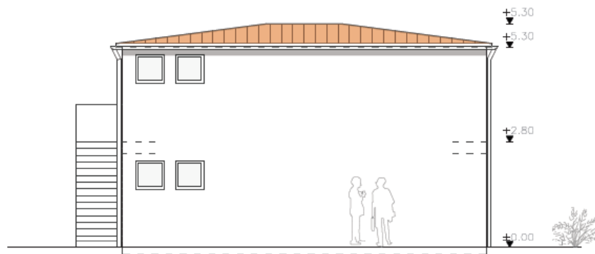
Seitenansicht A
