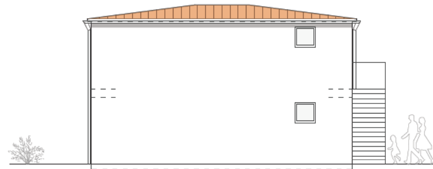
Seitenansicht B
